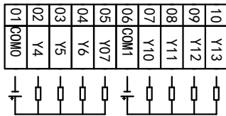
4.3寸一体机MC-20MR-6MT-430A-JK3U-E接线图
