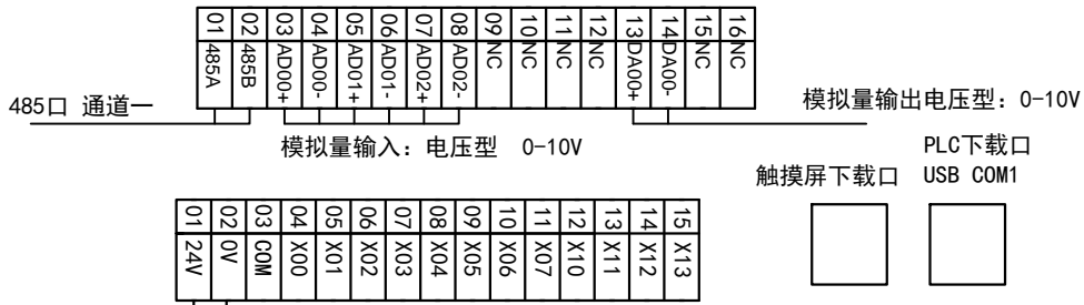
4.3寸一体机MC-20MR-6MT-430A-JK3U-E接线图
