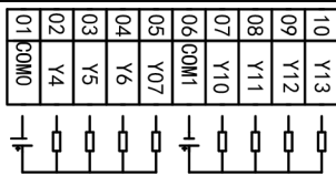
4.3寸一体机MC_20MR_6MT_F430A_FX_A接线图
