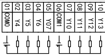
4.3寸一体机MC_20MR_6MT_FE430A_FX_A接线图
